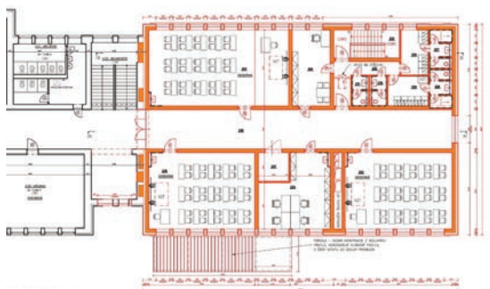
Půdorys přístavby 2 NP
