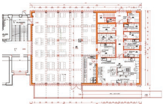
Půdorys přístavby 1 NP
